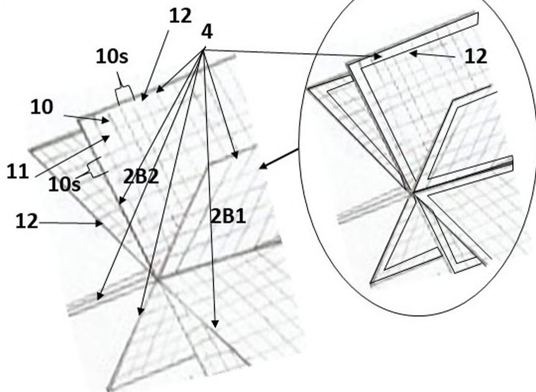
Figura 16. Se muestra en una perspectiva y con su detalle, los módulos de las mallas en "V" (2B1) y (2B2), ejemplificando algunas de las zonas en donde se dispone el resorte integrado (4), la zona de segmento (10s) del resorte integrado (4) y la trama (10) con su urdimbre (11)
