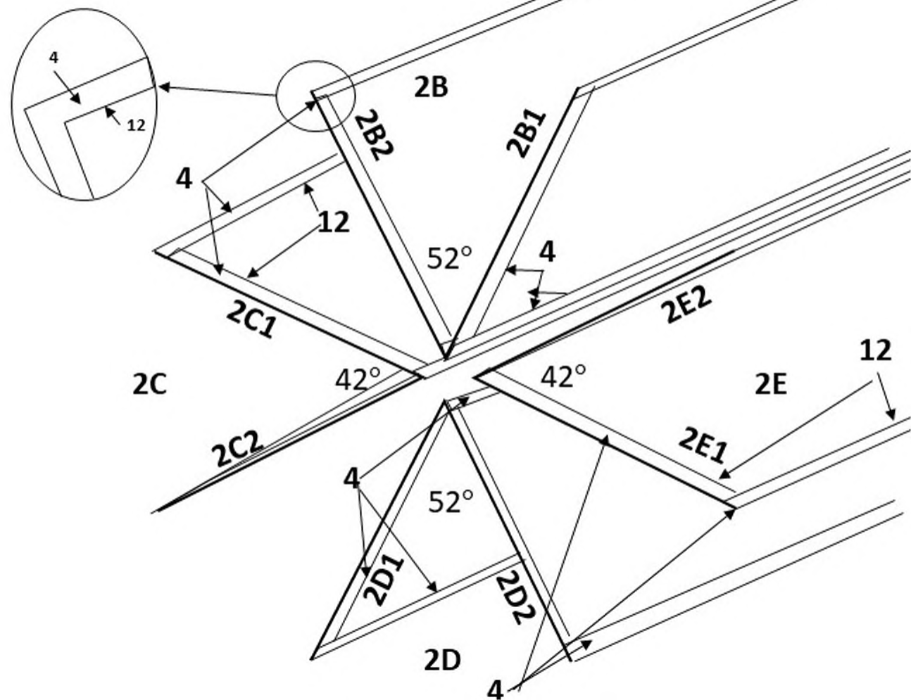
Figura 17. Se muestran en perspectiva los cuatro cuerpos de las mallas en "V" (2B), (2C), (2D) y (2E) con sus secantes (2B1), (2B2), (2C1), (2C2), (2D1), (2D2), (2E1) y (2E2), y los ángulos de 52° y 42°. Se muestran las zonas de ubicación de los resortes integrados (4). Se muestra un detalle con la ubicación de la línea de ubicación de segmentos (12) y del resorte integrado (4).
