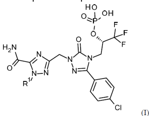
Fórmula (I)
