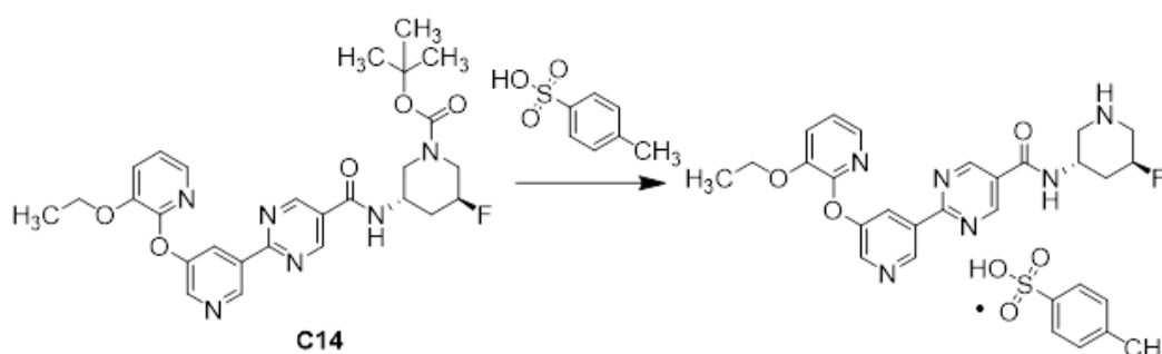
4, sal de p-toluensulfonato
