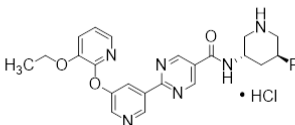
4, sal de clorhidrato
