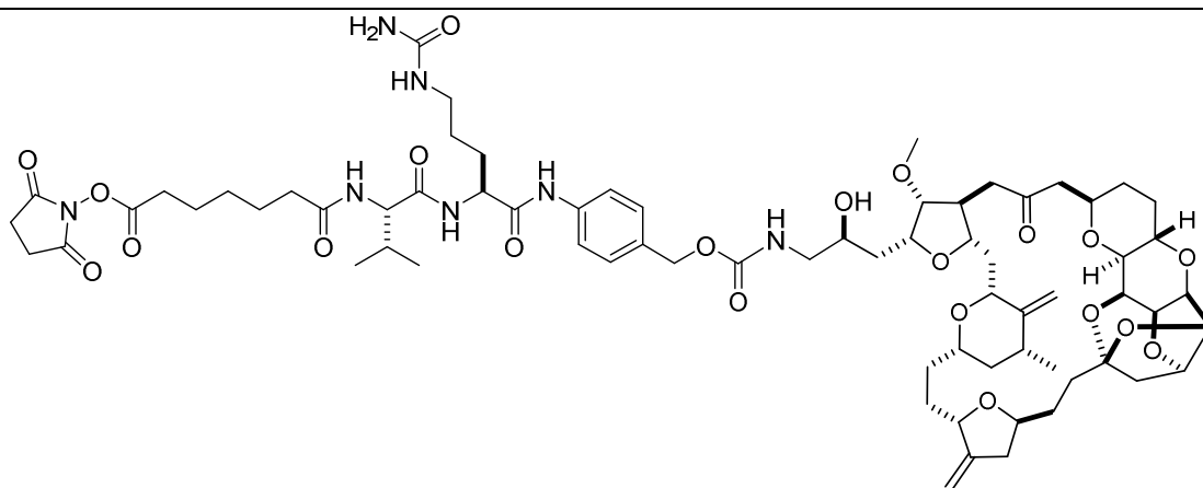
NHS-(CH 2 ) 5 -Val-Cit-PAB-eribulina (ER-001236941)
