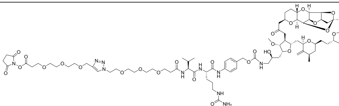
NHS-PEG3-triazol-PEG3-Val-Cit-PAB-eribulina (ER-001243700)
