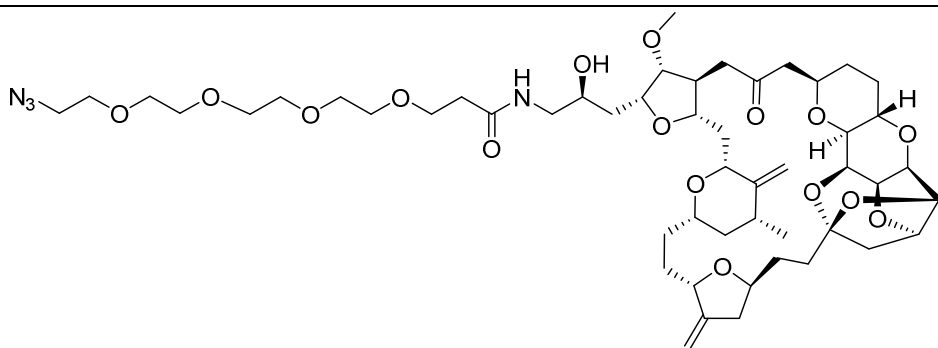
Azido-PEG4-eribulina
