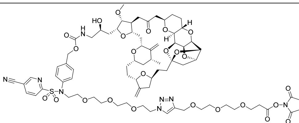
NHS-PEG3-triazol-PEG3-sulfonamida-PAB-eribulina (ER-001244623)
