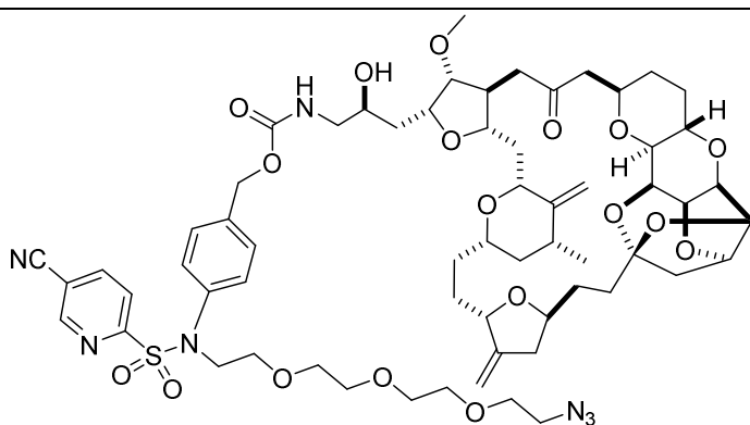
Azida-PEG3-sulfonamida-PAB-eribulina (ER-001138856)
