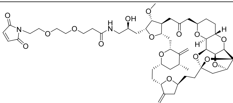
Mal-PEG2-eribulina
