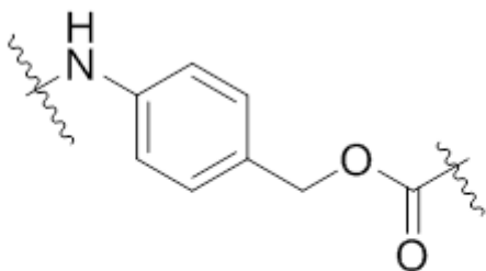
p-aminobenciloxycarbonilo
