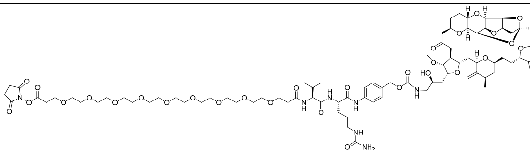
NHS-PEG9-Val-Cit-PAB-eribulina (ER-001242288)
