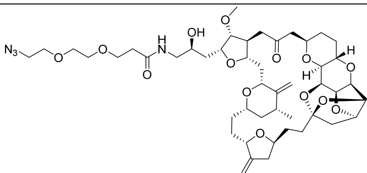
Azido-PEG2-eribulina
