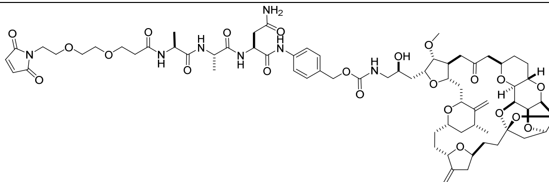
Mal-PEG2-Ala-Ala-Asn-PAB-eribulina (ER-001231679)
