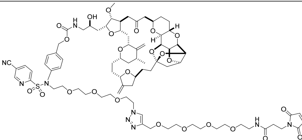
Mal-PEG4-triazol-PEG3-sulfonamida-PAB-eribulina (ER-001237505)
