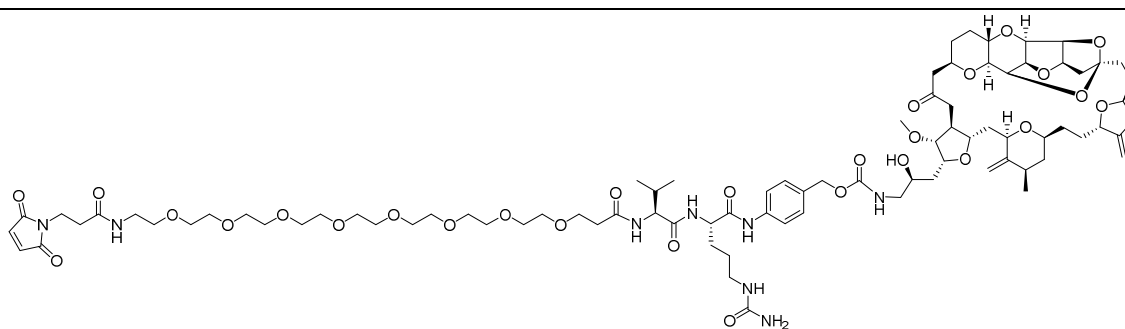
Mal-PEG8-Val-Cit-PAB-eribulina (ER-001242287)
