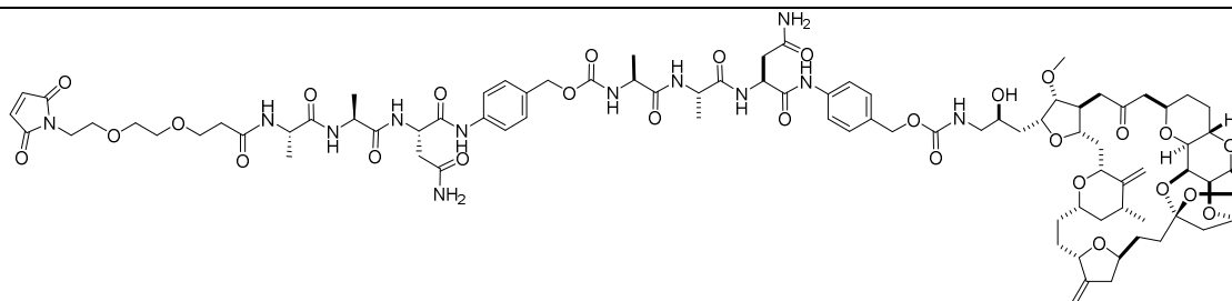
Mal-PEG2-Ala-Ala-Asn-PAB-eribulina (ER-001231679)
