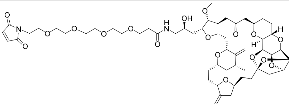
Mal-PEG4-eribulina
