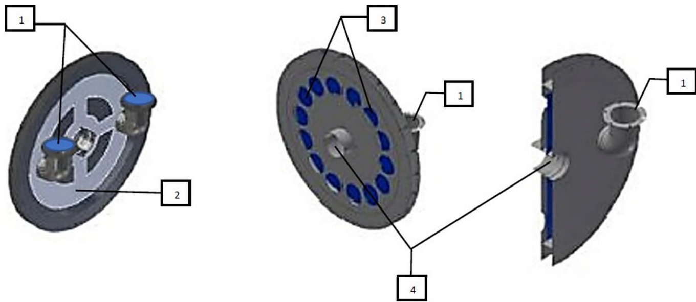
Figura_1 (Pre cámara de combustión)
