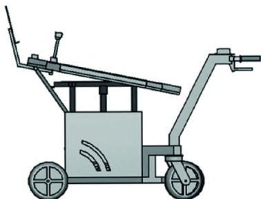
Posición plataforma inclinada
