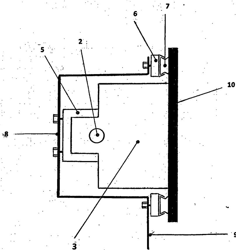
FIGURA 2 VISTA LATERAL
