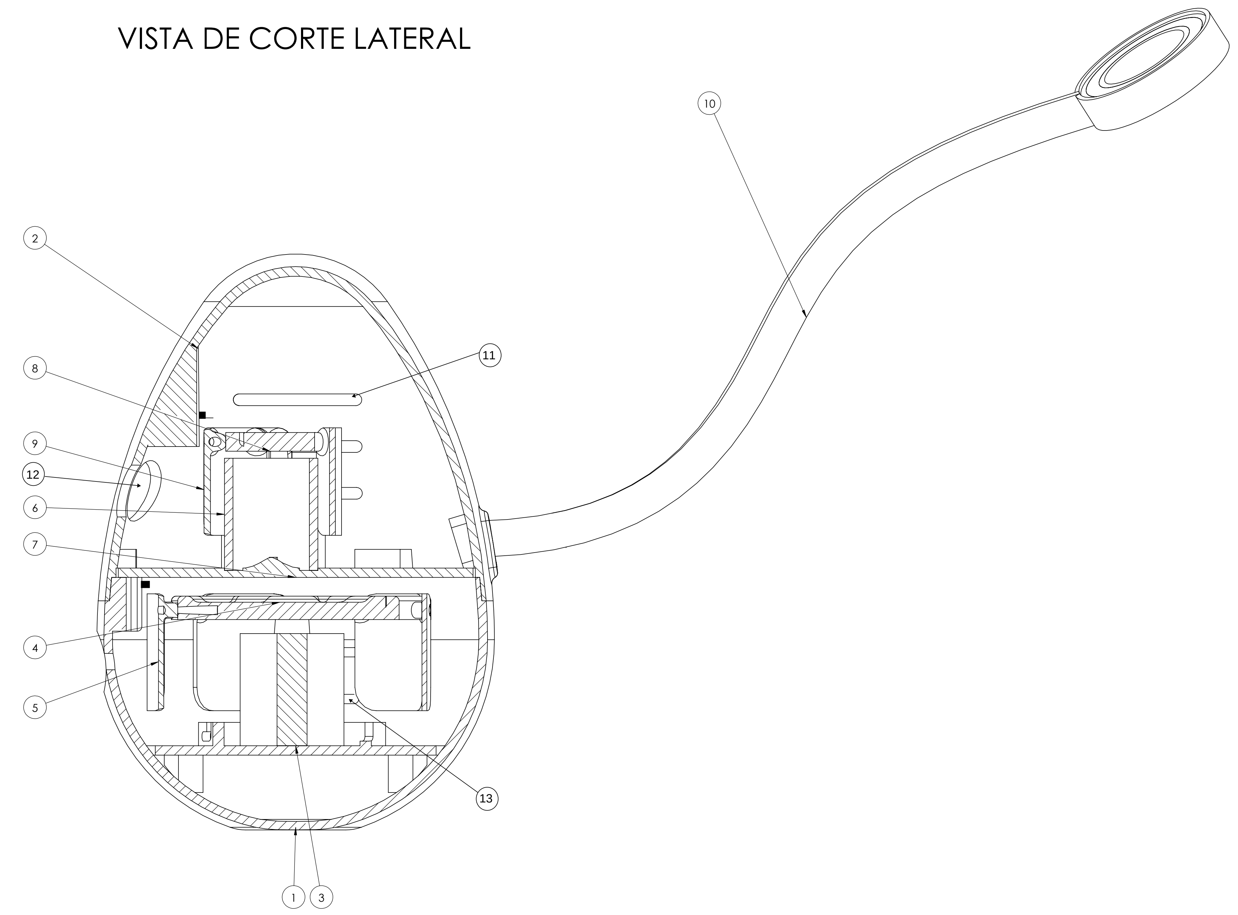
SECCIÓN A-A ESCALA 2:1
