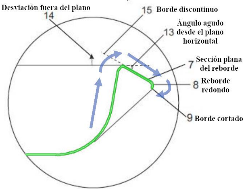
FIG. A. Esquema correspondiente a la presente invención. El color resaltado en verde corresponde a una vista de corte del perfil de la bandeja. Las flechas azules indican las direcciones y dobleces de la bandeja.
