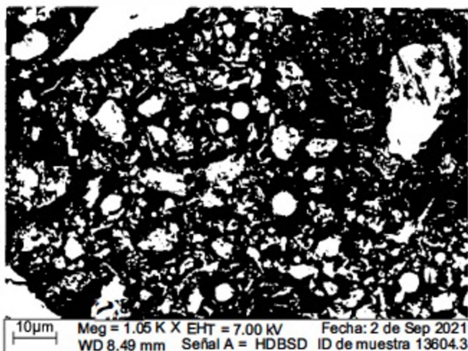
FIGURA 6: Ceniza de Vertedero Procesada a 1,05 KX de aumento
