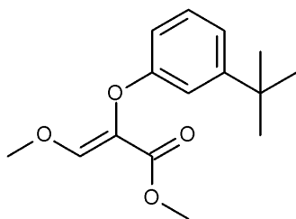
methyl (Z)-2-(3-tert-butylphenoxy)-3-methoxy-prop-2-enoate
