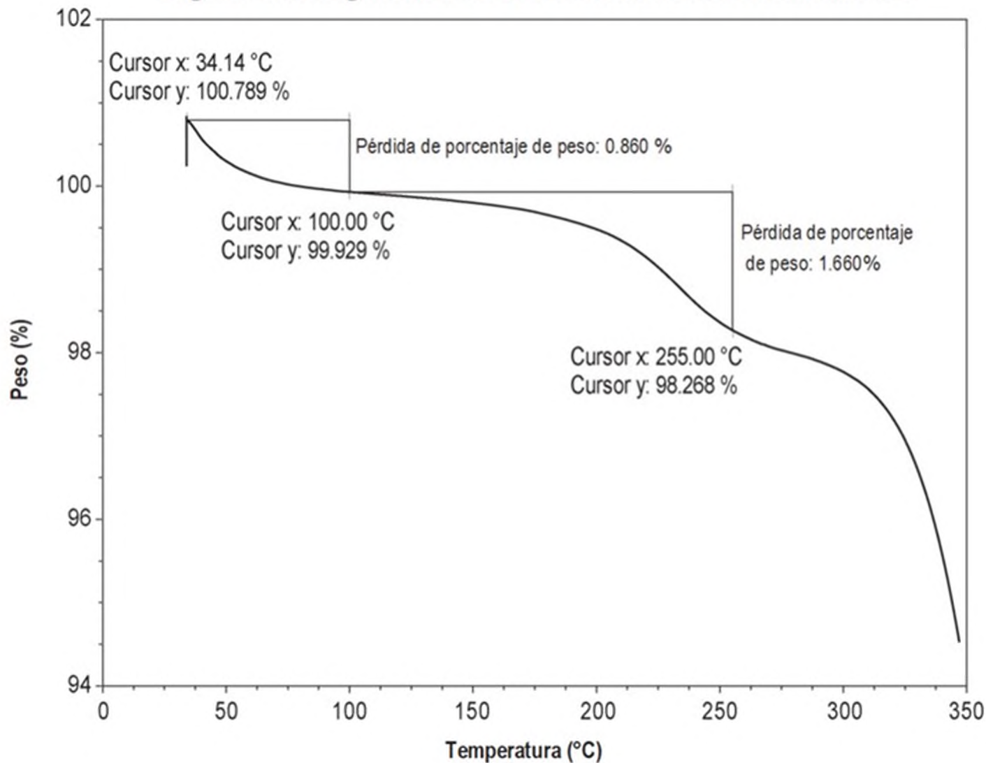
Fig. 10 Termograma de TGA de Patrón de Forma Libre D
