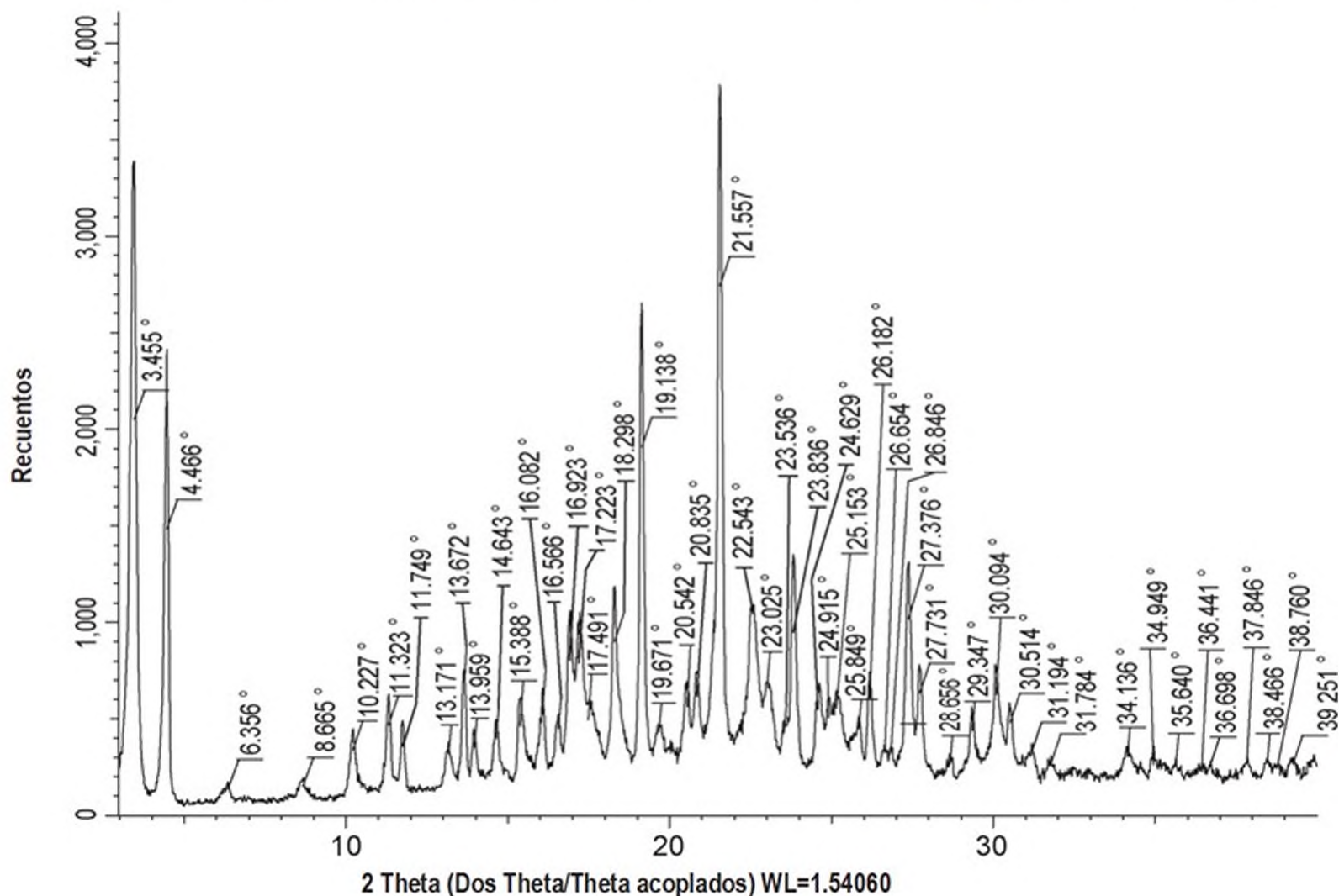
Figura 8A Patrón XRPD de Patrón de Forma Libre J (Compuesto A, Forma J)
