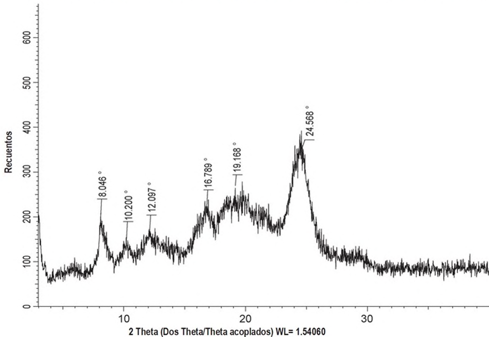
Figura 7 A Patrón XRPD de Patrón de Forma Libre G (Compuesto A, Forma G)
