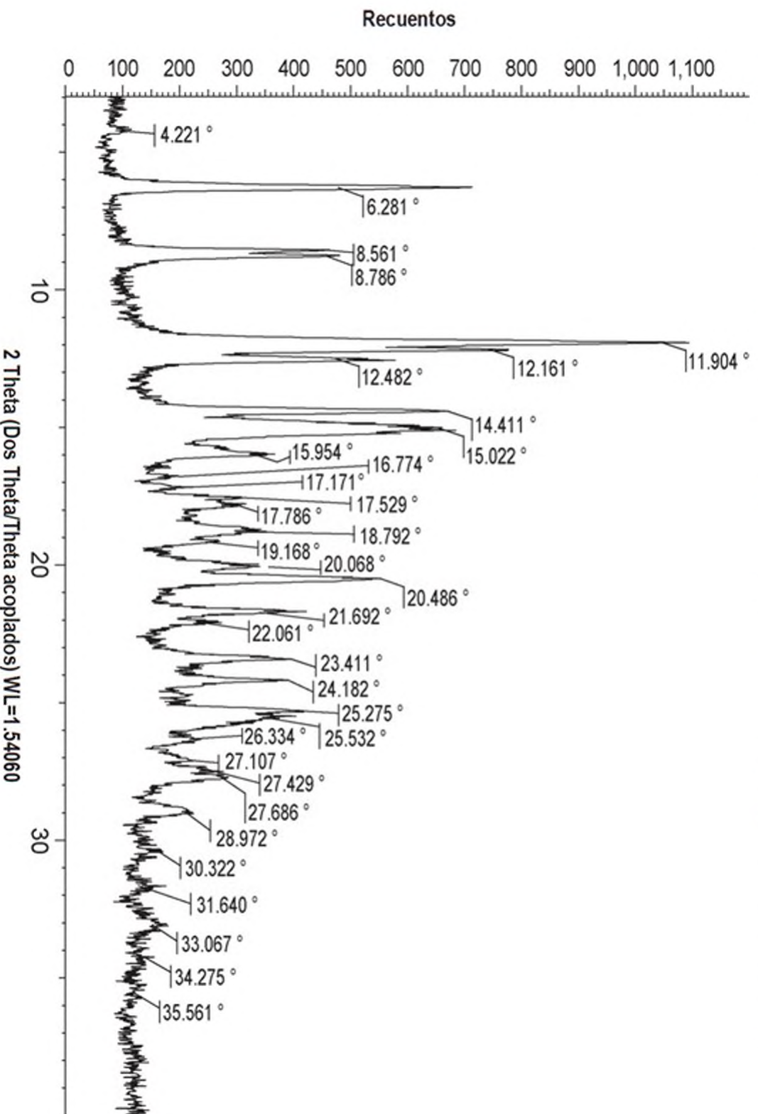
Figura 6A Patrón XRPD de Patrón de Forma Libre F (Compuesto A, Forma F)
