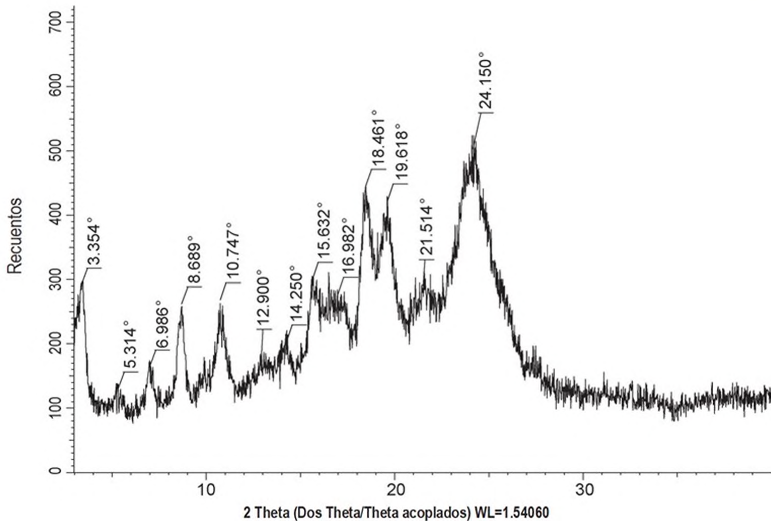
Figura 4A Patrón XRPD de Patrón de Forma Libre D (Compuesto A, Forma D)
