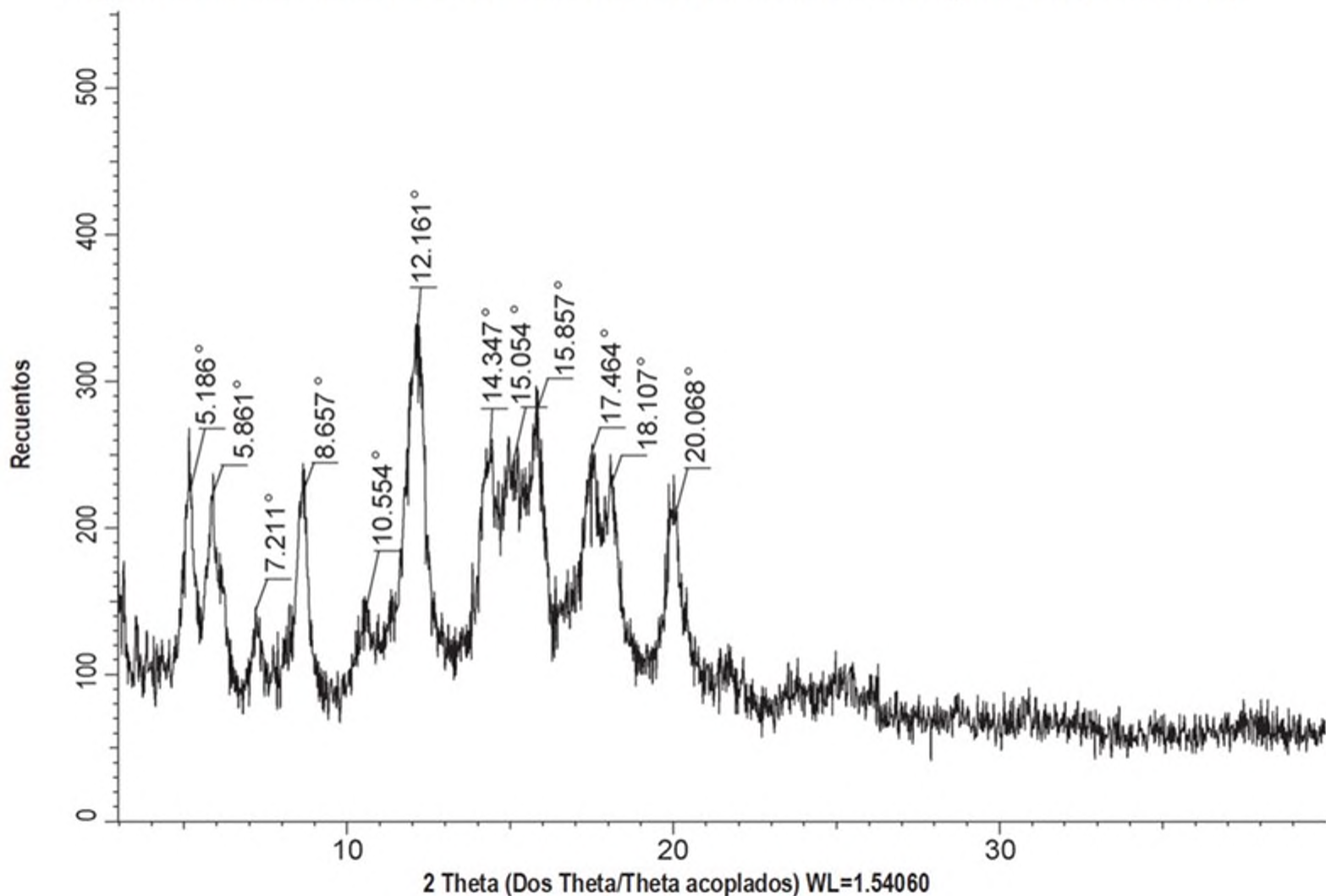
Figura 3A Patrón XRPD de Patrón de Forma Libre C (Compuesto A, Forma C)
