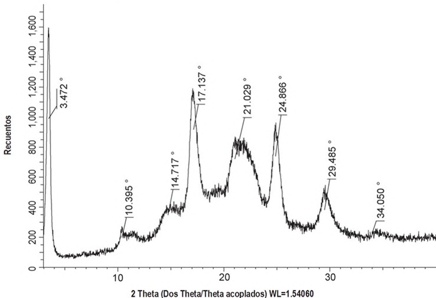
Figura 1A Patrón XRPD del Patrón de Forma Libre A (Compuesto A, Forma A)
