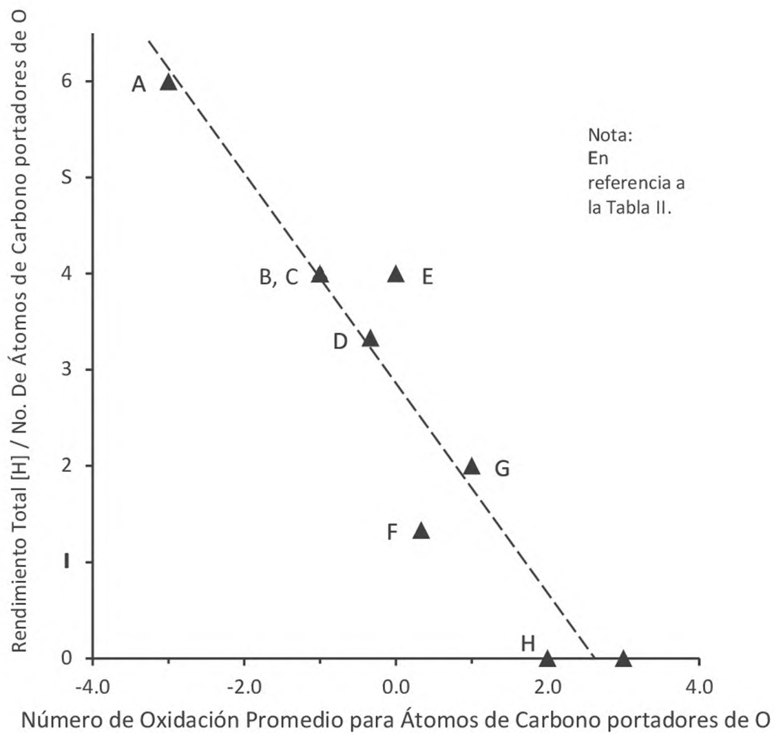
FIGURA 7. [H] Rendimiento vs Número de Oxidación Promedio para Átomos de Carbono en A2.
