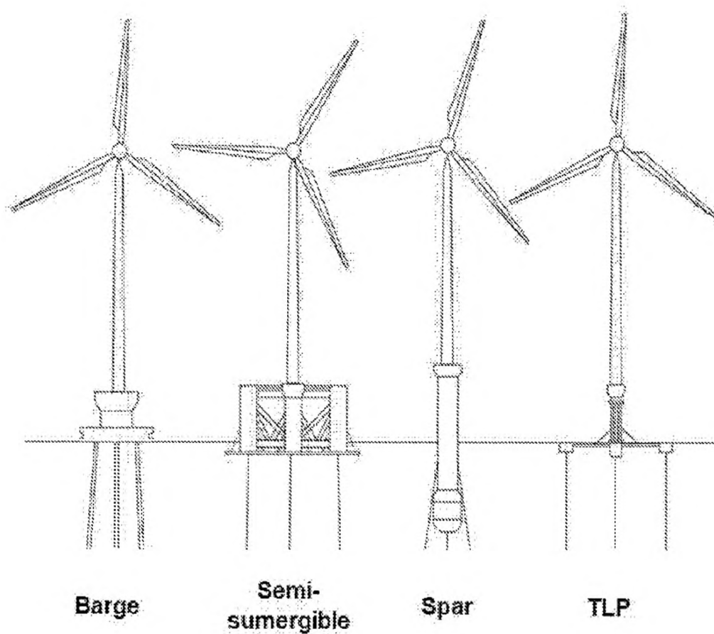
FIG. 1 (TÉCNICA ANTERIOR)
