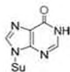
Inosina I
