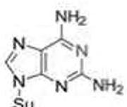
2,6- Diaminopurina DAP
