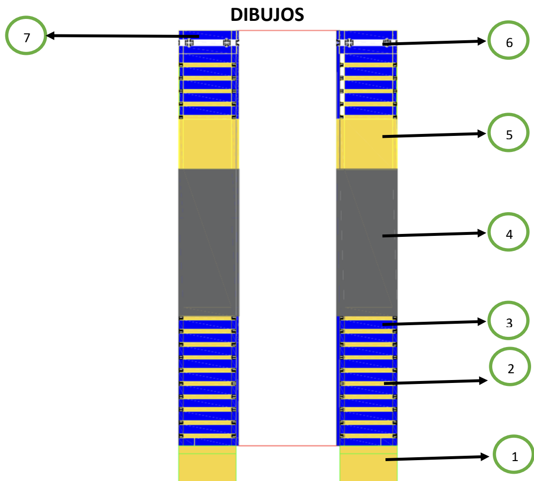
FIGURA N. 1 INVENCION – TOPE RUEDA DE SEGURIDAD DE PARQUEO VISTA DESDE ARRIBA (COMPONENTES)
