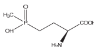
L-glufosinato
