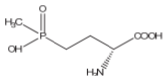
D-glufosinato
