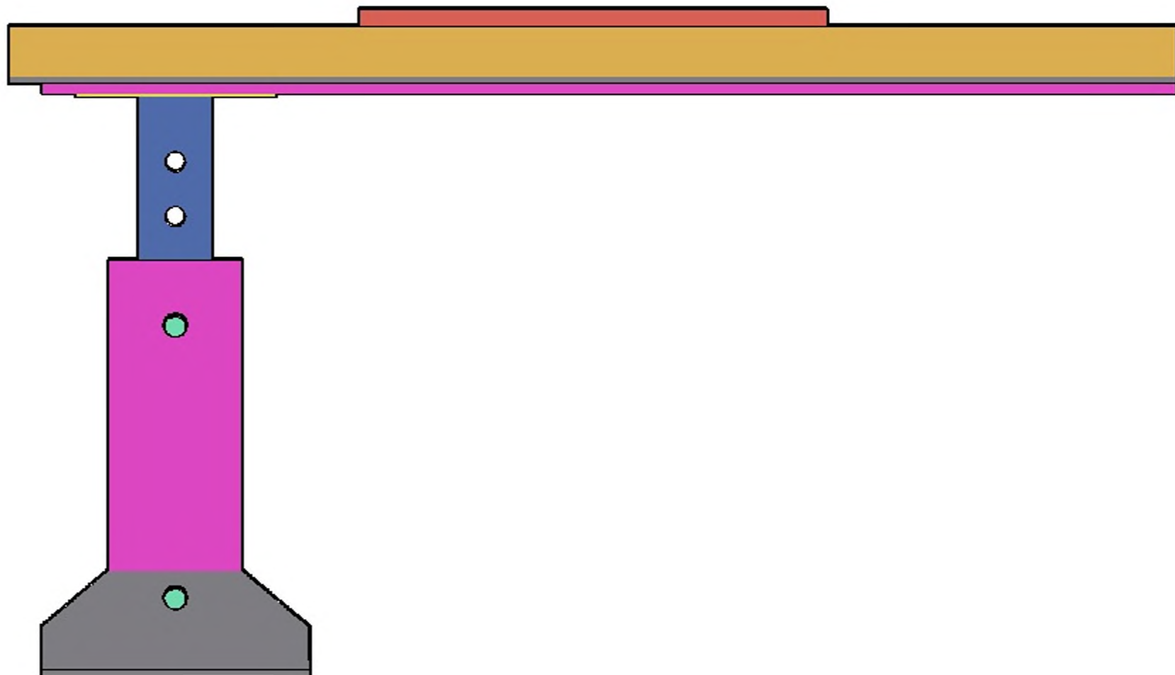
Vista lateral
