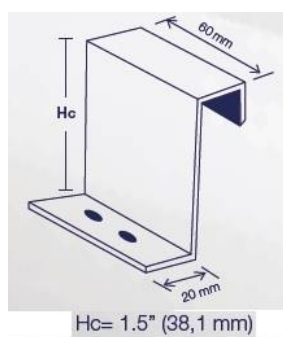
FIGURA 3: Muestra los elementos de fijación para la teja Traslapolsofoam
