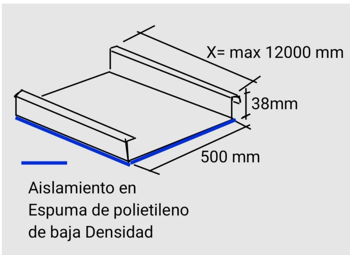
FIGURA 2: Muestra Isometría de la teja Traslapolsofoam
