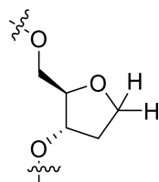
Fórmula (IIa').
