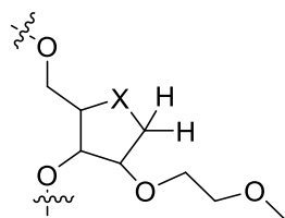
Fórmula (III)
