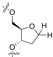
Fórmula (IIa').
