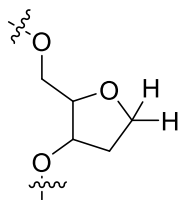
Fórmula (IIa).
