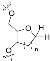
Fórmula (Ia)
