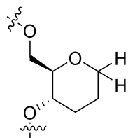
Fórmula (IIIa').
