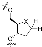
Fórmula (II')
