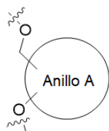
5 Fórmula (X)
