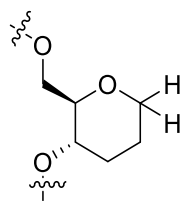
Fórmula (IIIa').
