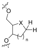
Fórmula (I)
