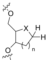
Fórmula (I)
