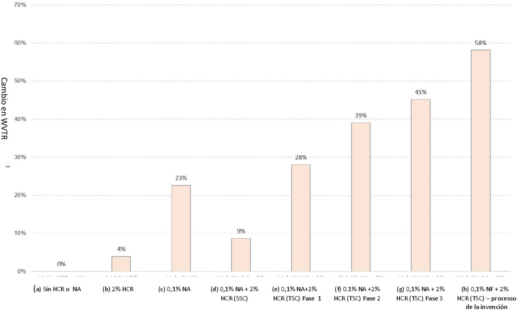
Efecto sobre WVTR utilizando diferentes procesos
