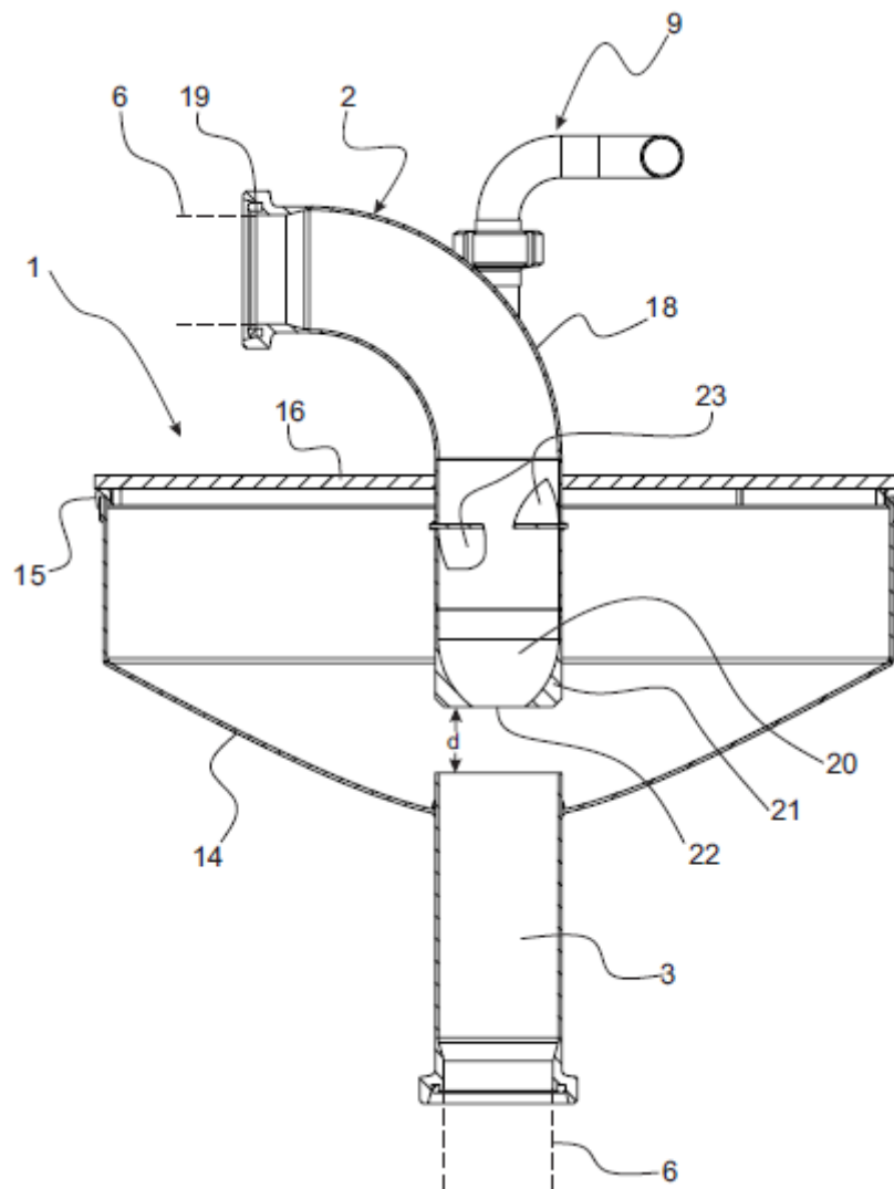
Fig. 7 C-C Corte
