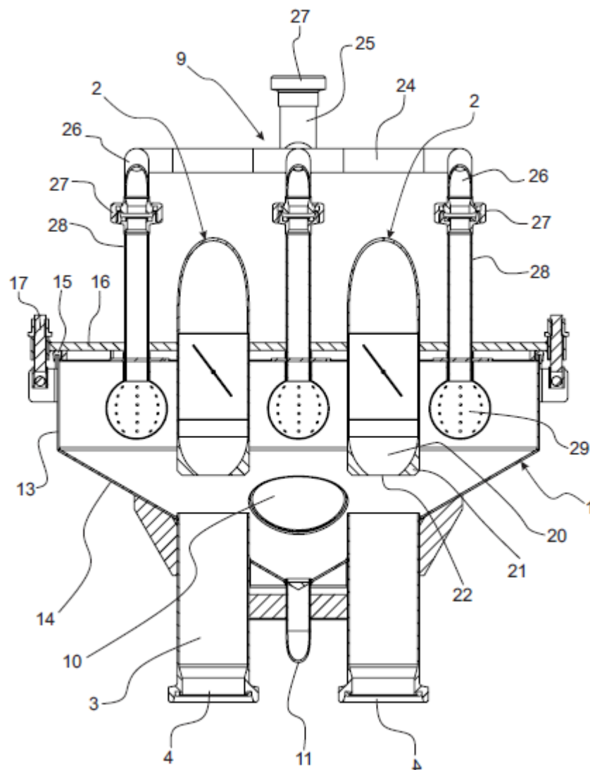
Fig. 4 A-A Corte
