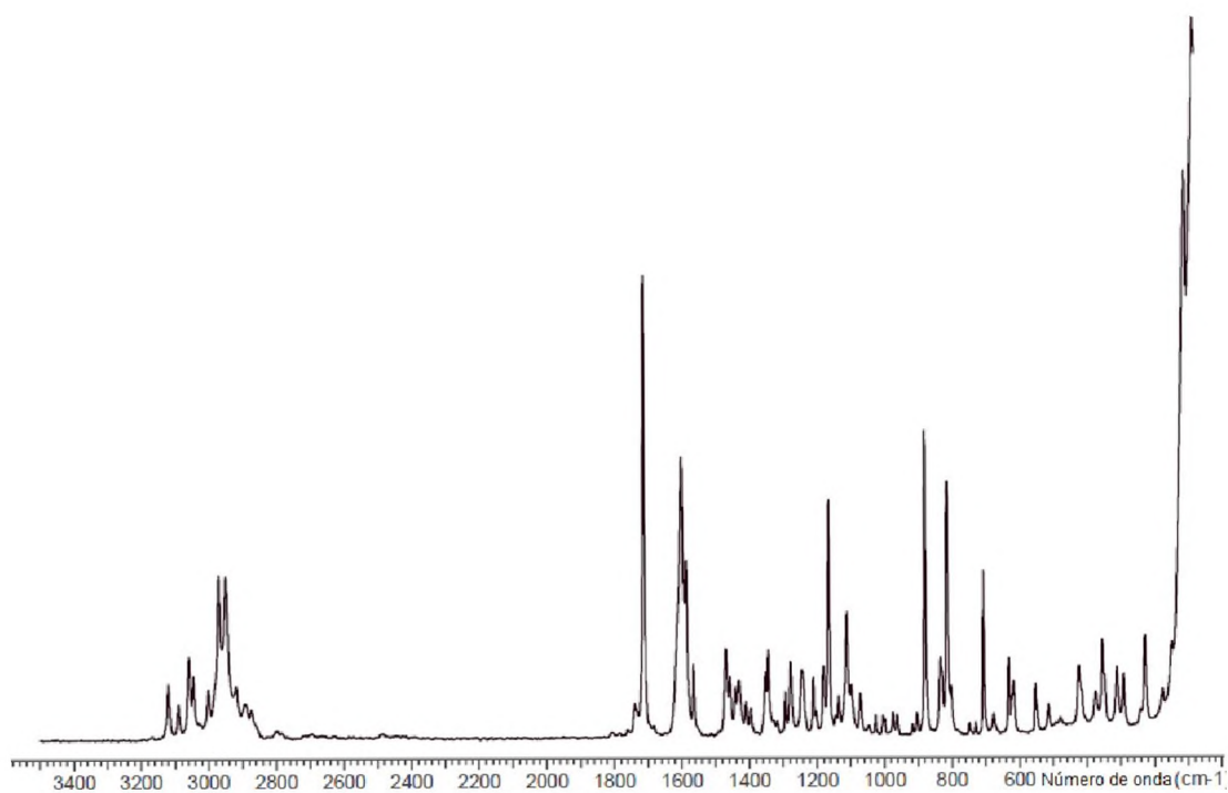
Fig. 1b: Espectro FT Raman de la forma polimórfica A de 4-[(6-cloro-3-piridilmetil)(2,2-difluoretil)amino]furan-2(5H)-ona
