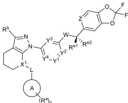
(I–a)
