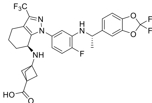
Ácido 3-[[[(7R)-1-[3-[[[(1S)-1-(2,2-difluoro-1,3-benzodioxol-5-il)etil]amino]-4-fluoro-fenil]-3-(trifluorometil)-4,5,6,7-tetrahidroindazol-7-il]amino]biciclo[1.1.1]pentano-1-carboxílico
