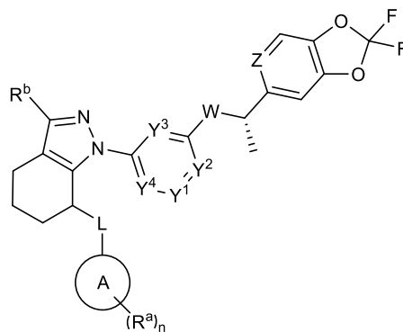
(I-a2)
