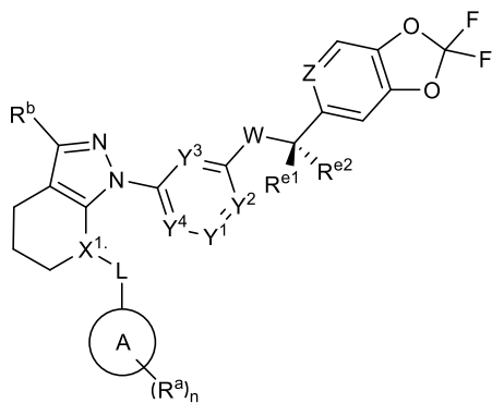
(I-a)
