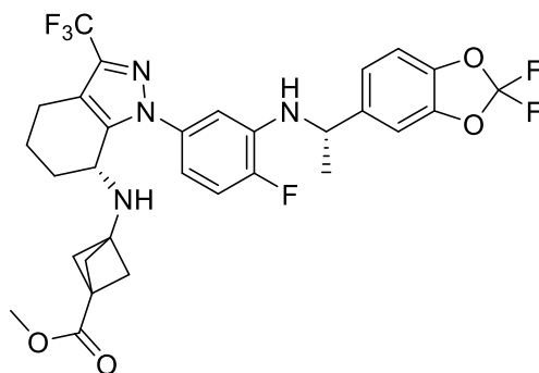
Ácido 3-[[[(7R)-1-[3-[[[(1S)-1-(2,2-difluoro-1,3-benzodioxol-5-il)etil]amino]-4-fluoro-fenil]-3-(trifluorometil)-4,5,6,7-tetrahidroindazol-7-il]amino]biciclo[1.1.1]pentano-1-carboxílico
