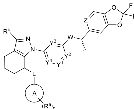
(I-a2)
