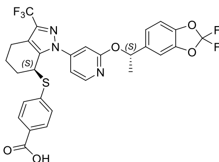
Ácido 4-[[[(7S)-1-[2-[(1S)-1-(2,2-difluoro-1,3-benzodioxol-5-il)etoxi]-4-piridil]-3-(trifluorometil)-4,5,6,7-tetrahidroindazol-7-il]sulfanil]benzoico
