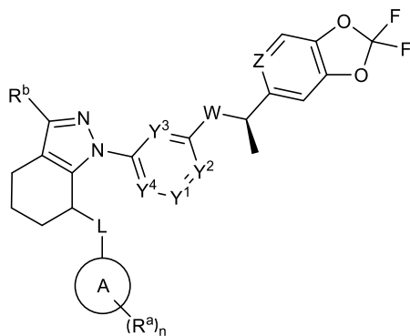
(I-a1)
