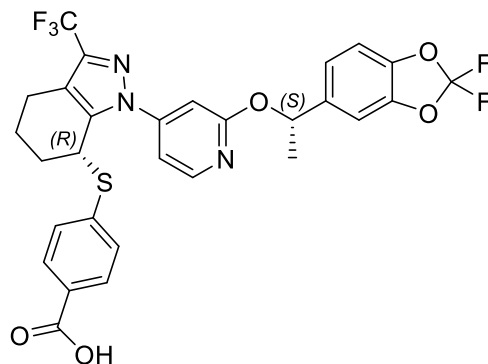
Ácido 4-[[[(7S)-1-[2-[(1S)-1-(2,2-difluoro-1,3-benzodioxol-5-il)etoxi]-4-piridil]-3-(trifluorometil)-4,5,6,7-tetrahidroindazol-7-il]sulfanil]benzoico
