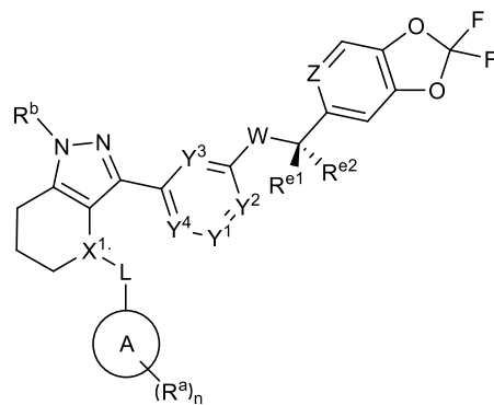
(II-a)
