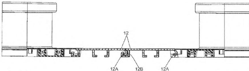
FIG. 4C CORTE B.B
