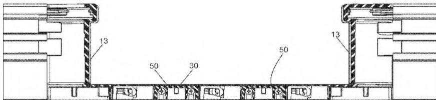
FIG. 4C CORTE B.B
