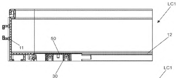
FIG. 5C CORTE C.C
