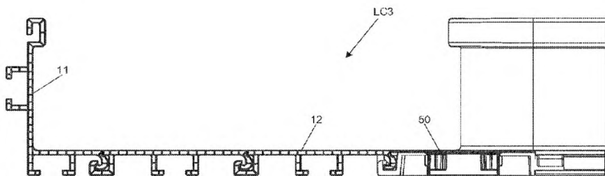
FIG. 6C CORTE E.E
