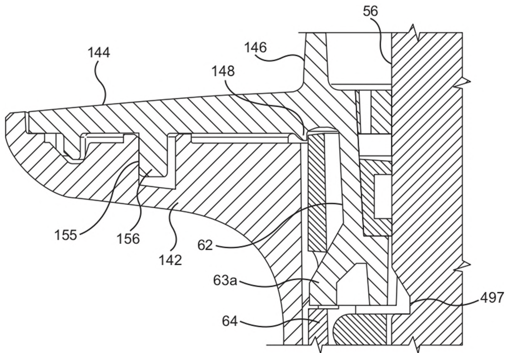
FIG. 54A
